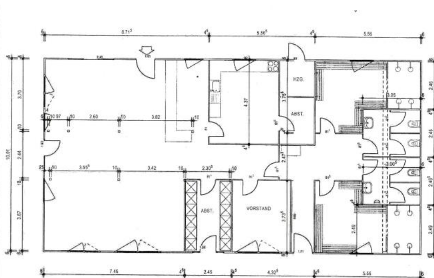
UMBAU TC GENSSINGEN -VARIANTE 2- M. 1:100 27.09.2017
